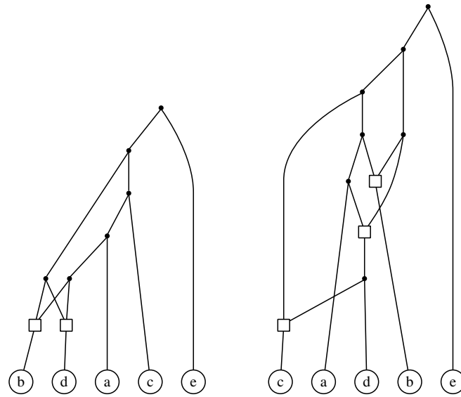
Рис. 1.2: Возможные гибридизационные сети, для деревьев из Рис. 1.1, с двумя и тремя ретикулярными событиями соответственно. Ретикулярные вершины обозначены квадратами.
