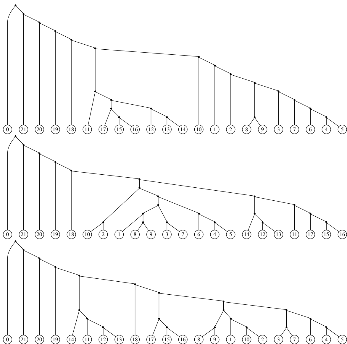
Рис. 1.3: Входные деревья для теста NdhfPhytRbcl.
