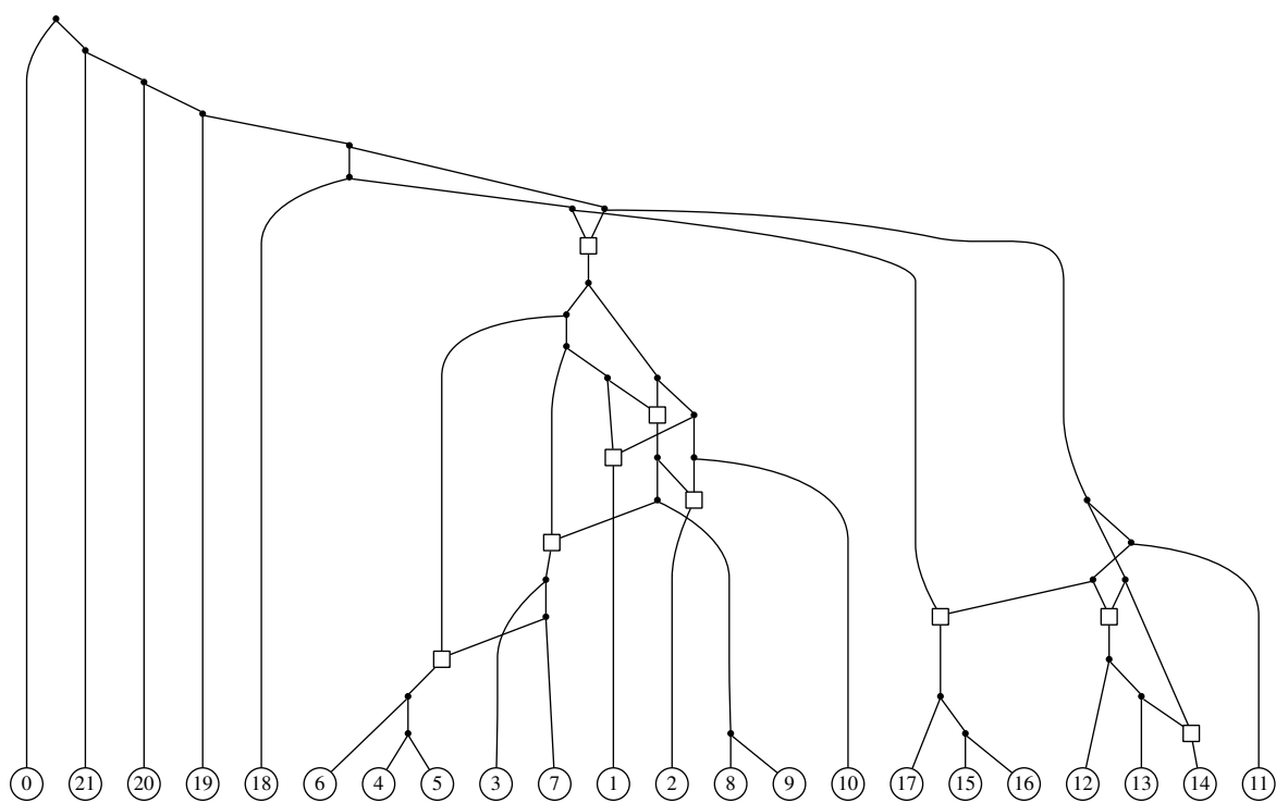
Рис. 1.4: Минимальная гибридизационная сеть для теста NdhfPhytRbcl.
