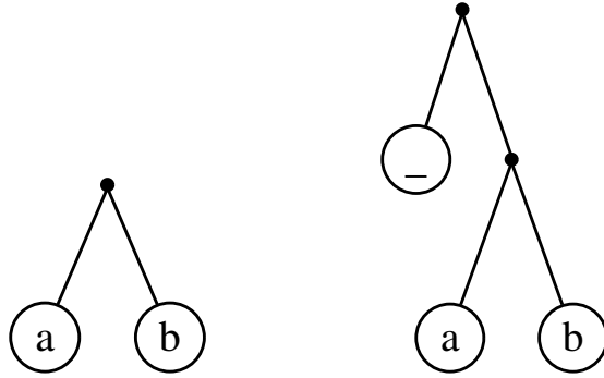
Рис. 2.1: Добавление фиктивного корня к дереву.
