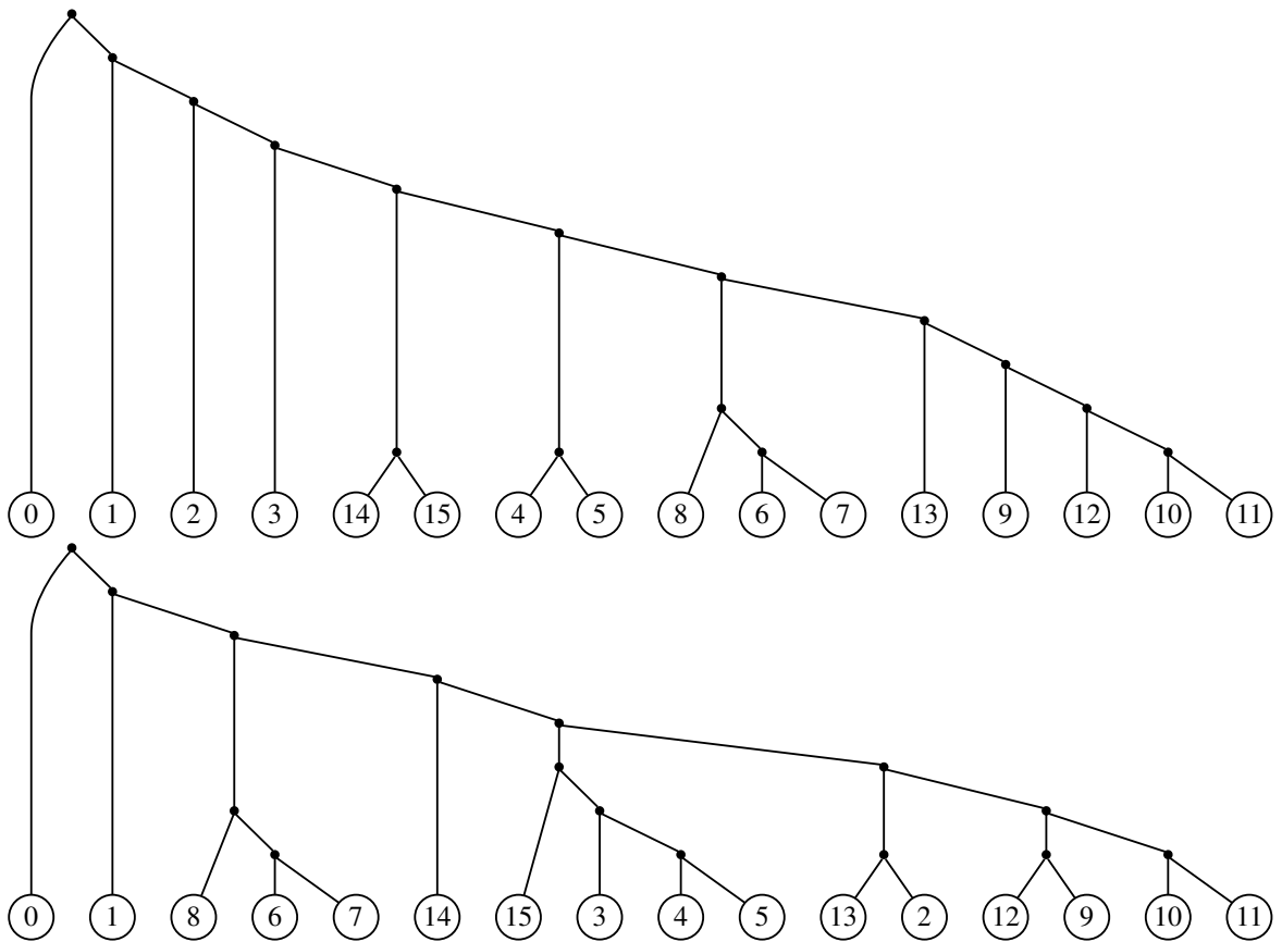
Рис. 1.1: Входные деревья для теста WaxyIts.
