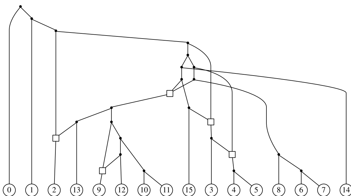
Рис. 1.2: Минимальная гибридизационная сеть для теста WaxyIts.
