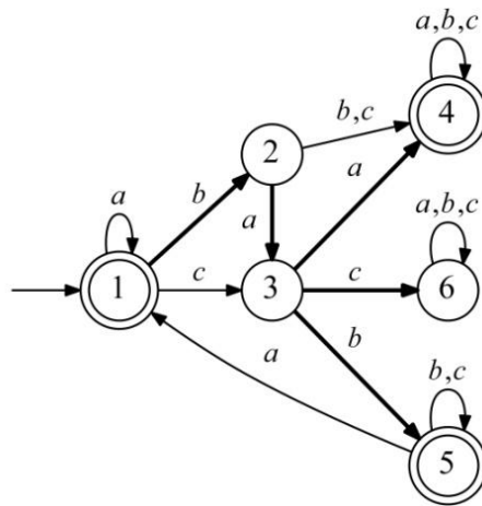
Рис. 4. Пример DFS-пронумерованного ДКА
