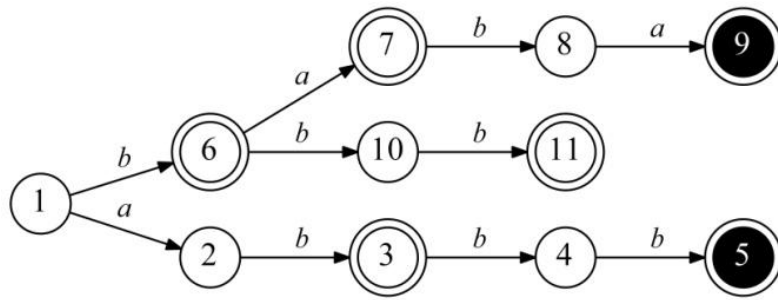
Рис. 2 Пример префиксного автомата
