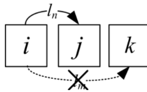
Рис. 8. Иллюстрация к предикатам, упорядочивающим состояния в алфавитном порядке. Если состояние i – это предок состояний j и k , l_n ( l_m ) – минимальные в алфавитном порядке символы на переходах между i и j ( i и k ), тогда l_m не может быть меньше чем l_n
