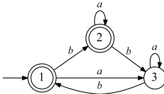
Рис. 6. Пример не DFS-пронумерованного ДКА
