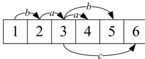
Рис. 5. Пример вспомогательного массива, построенного в ходе работы алгоритма DFS при обходе ДКА на рис. 4
