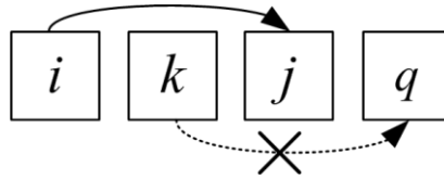
Рис. 7. Часть массива, иллюстрирующая предикаты упорядочивания родителей. Пунктиром показан переход, которого не должно быть в DFS-пронумерованном ДКА
