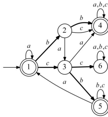
Рис. 9. Пример BFS-пронумерованного ДКА
