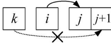
Рис. 11. Часть очереди, иллюстрирующая предикаты упорядочивания родителей. Пунктиром показан переход, который невозможен в BFS-пронумерованном ДКА
