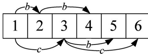
Рис. 10. Пример очереди, использованной в алгоритме BFS при обходе ДКА на рис. 8
